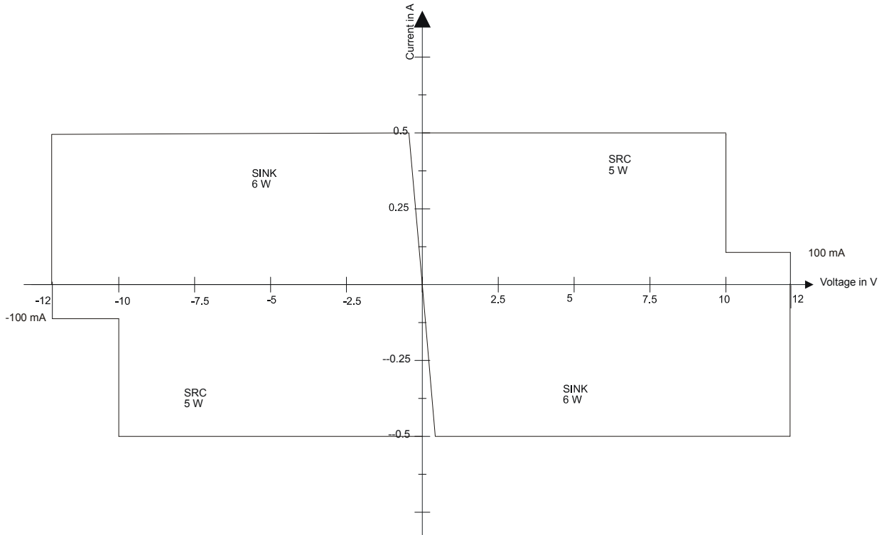
Bild 5-2 Strom-/Spannungskennlinie
