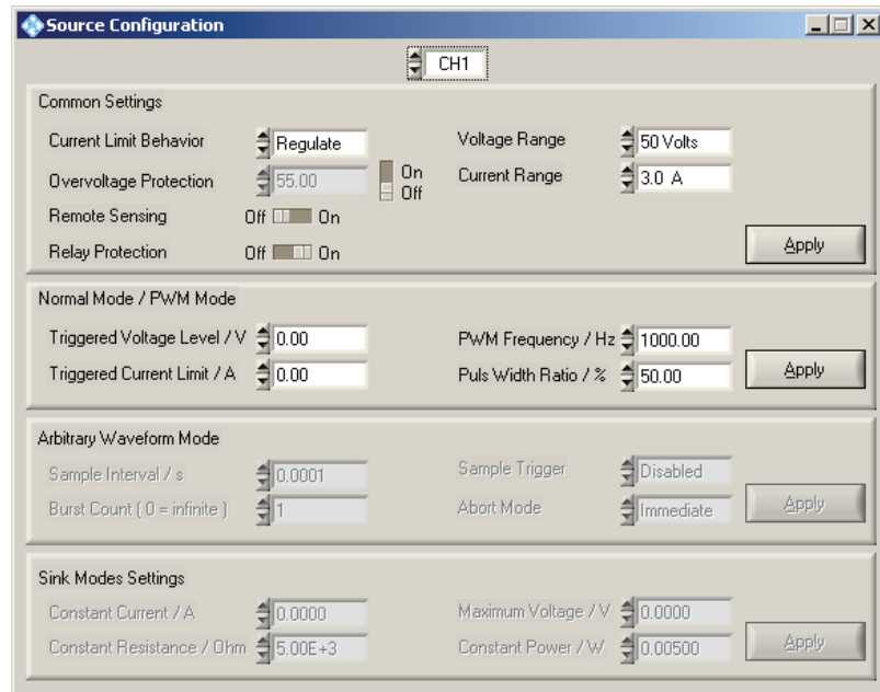
Bild 7-2 Konfiguration der Quellen
