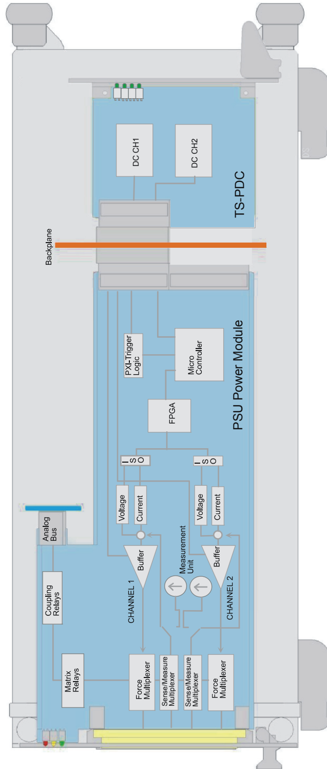
Bild 3-1 Funktionsblockschaltbild R&S TS-PSU12
