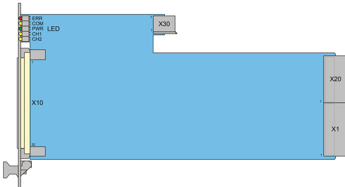
Bild 4-1 Anordnung der Steckverbinder und LEDs PSU-Powermodul
