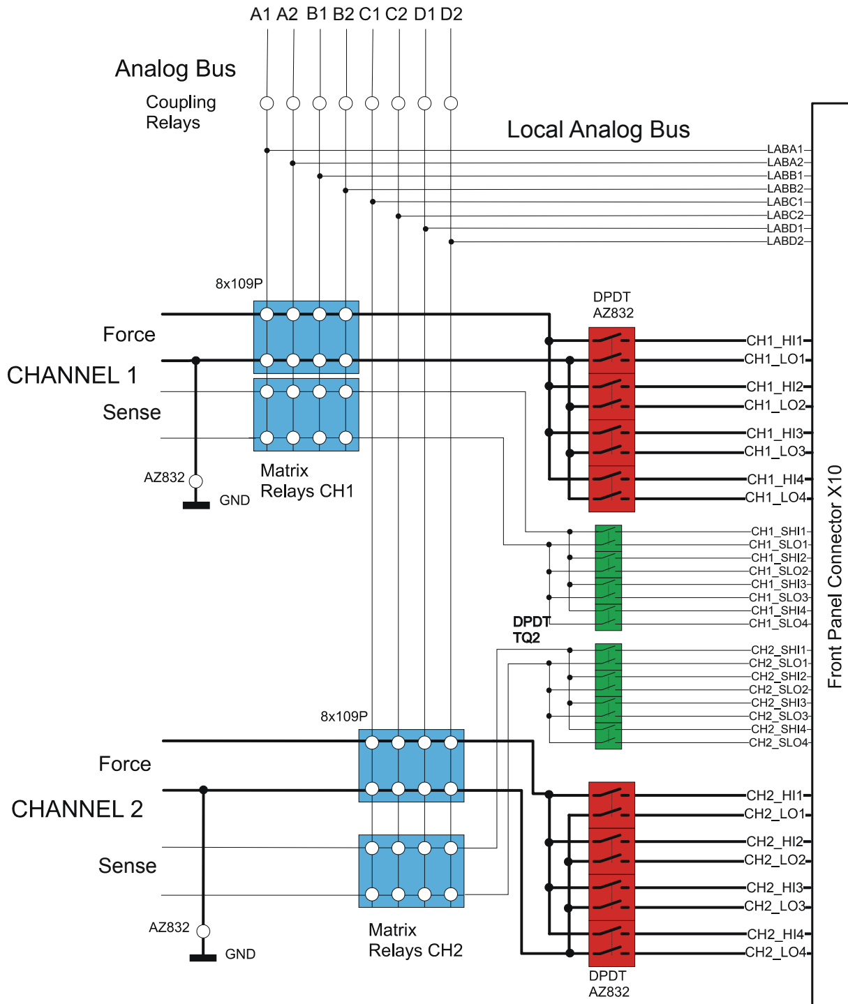
Bild 5-3 Signalverschaltung
